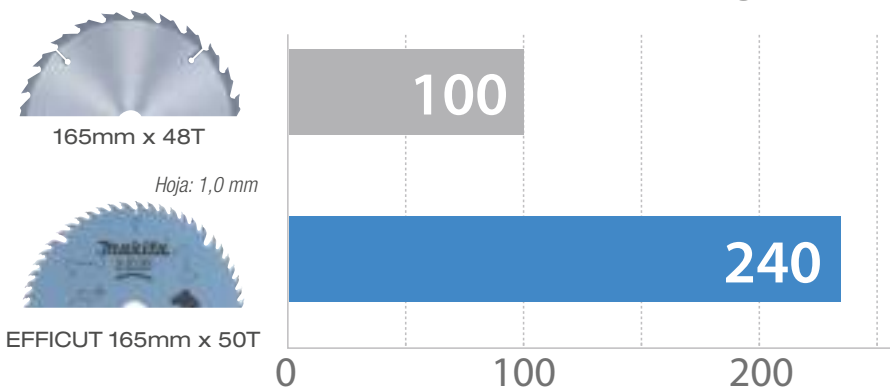
Hoja: 1,6 mm Cantidad de cortes con una carga
